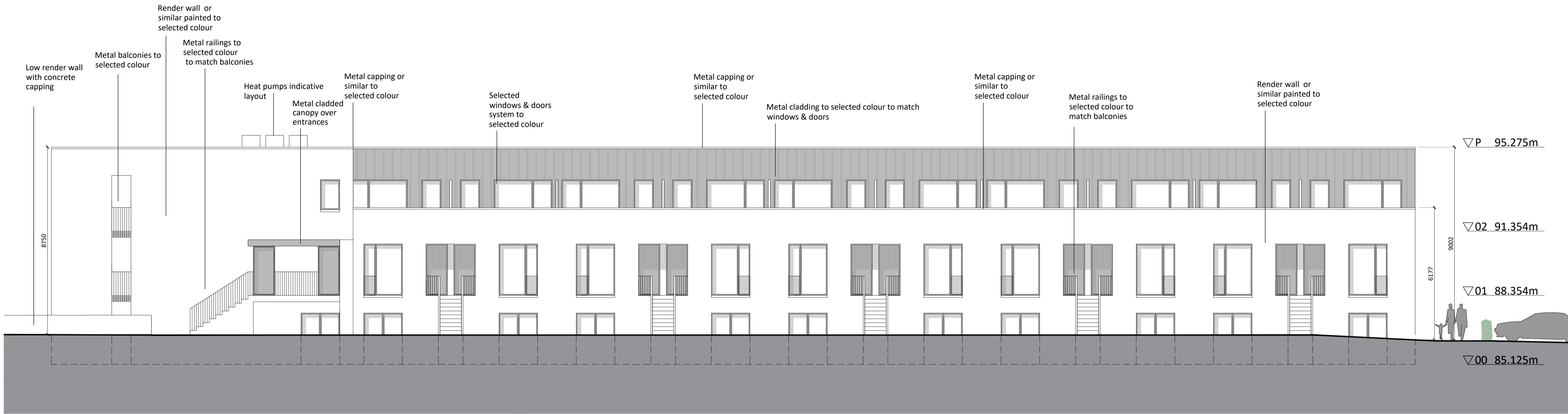
ELEVATION 1
