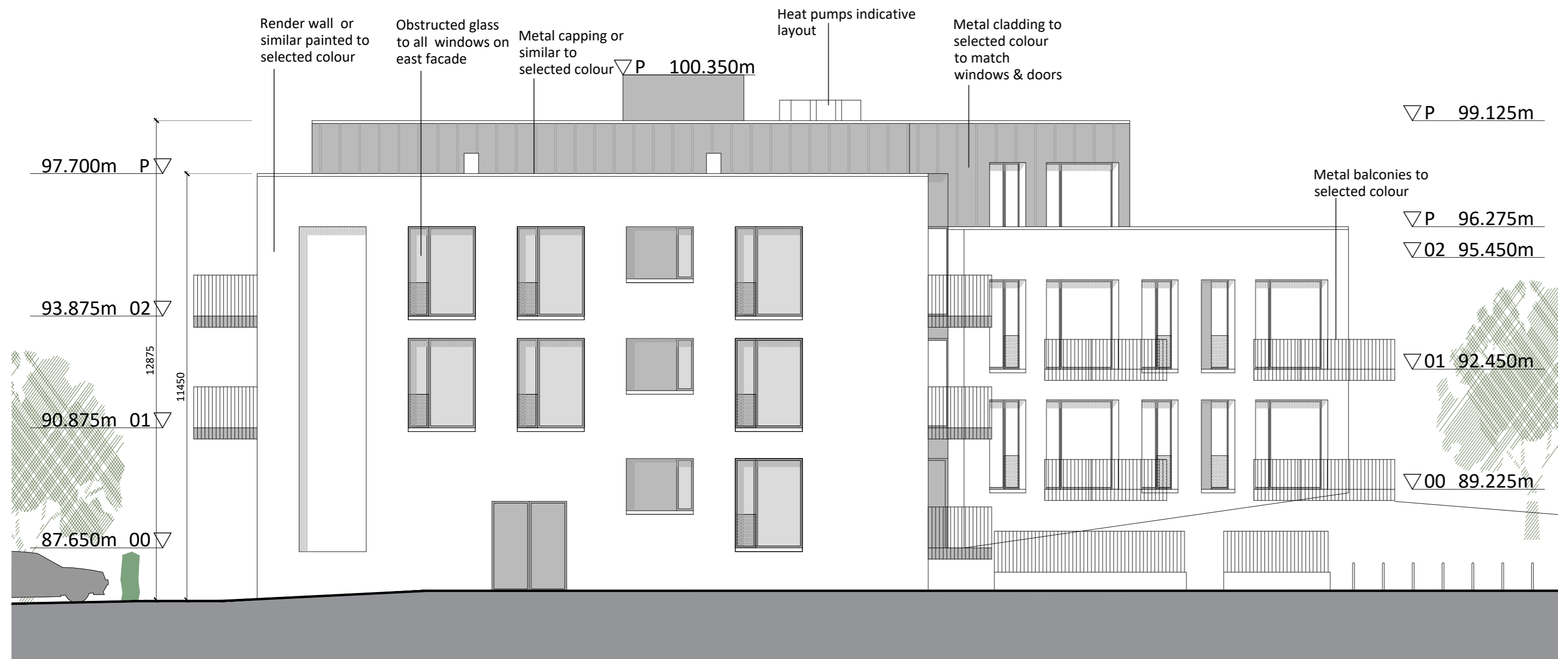
ELEVATION 1
