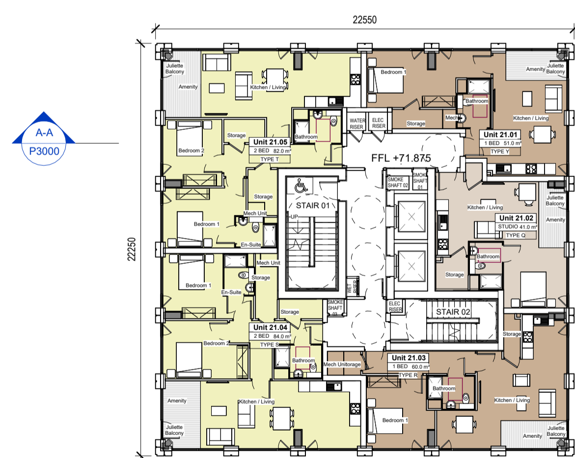
4 L21 FLOOR PLAN 1 : 200
