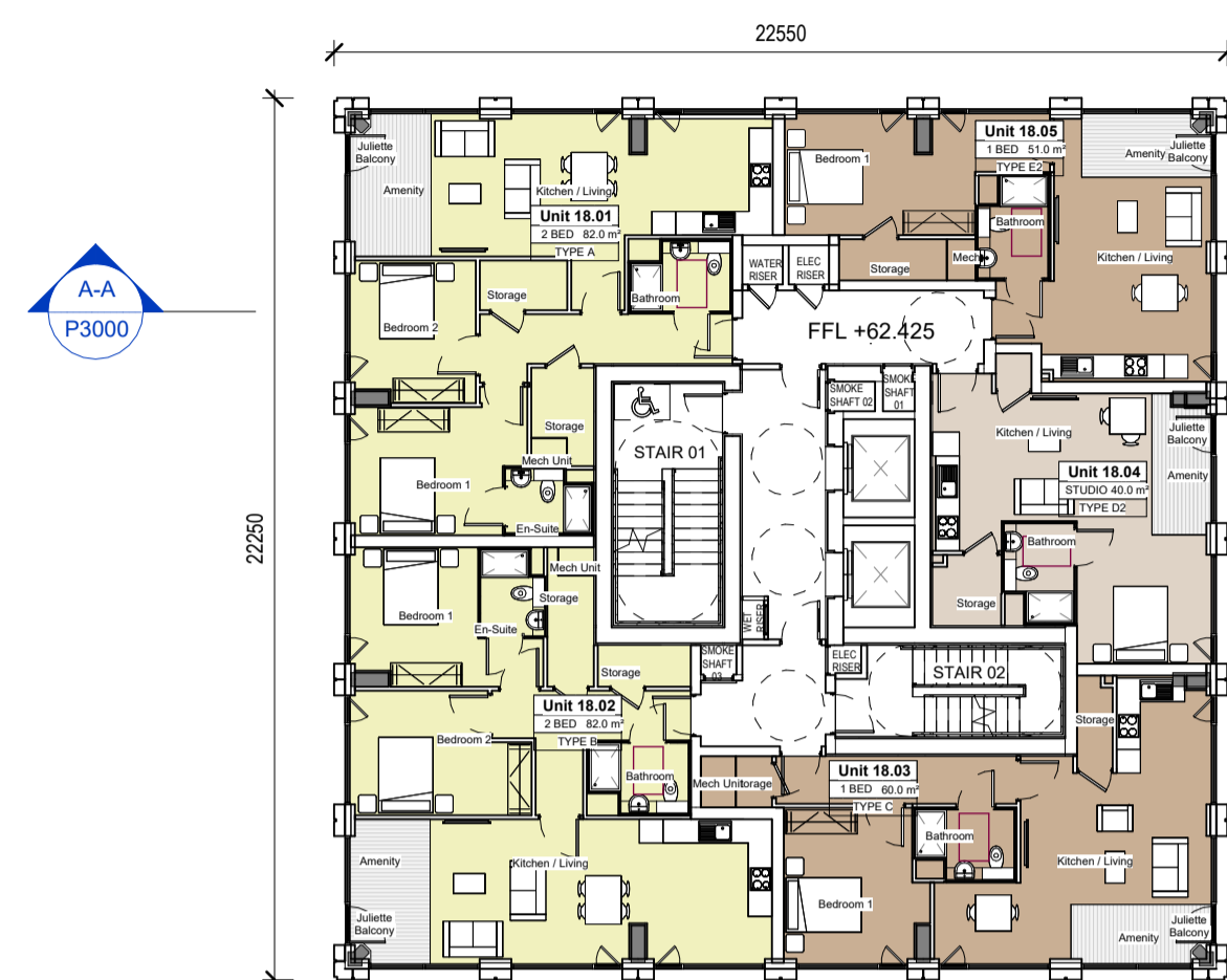
1 L18 FLOOR PLAN 1 : 200
