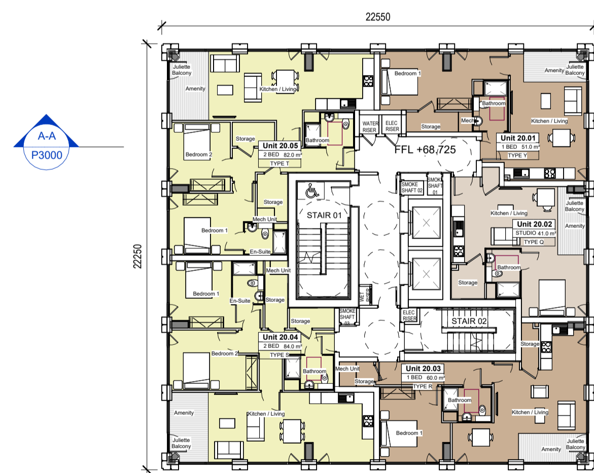
3 L20 FLOOR PLAN 1 : 200
