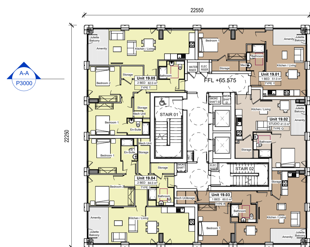
2 L19 FLOOR PLAN 1 : 200
