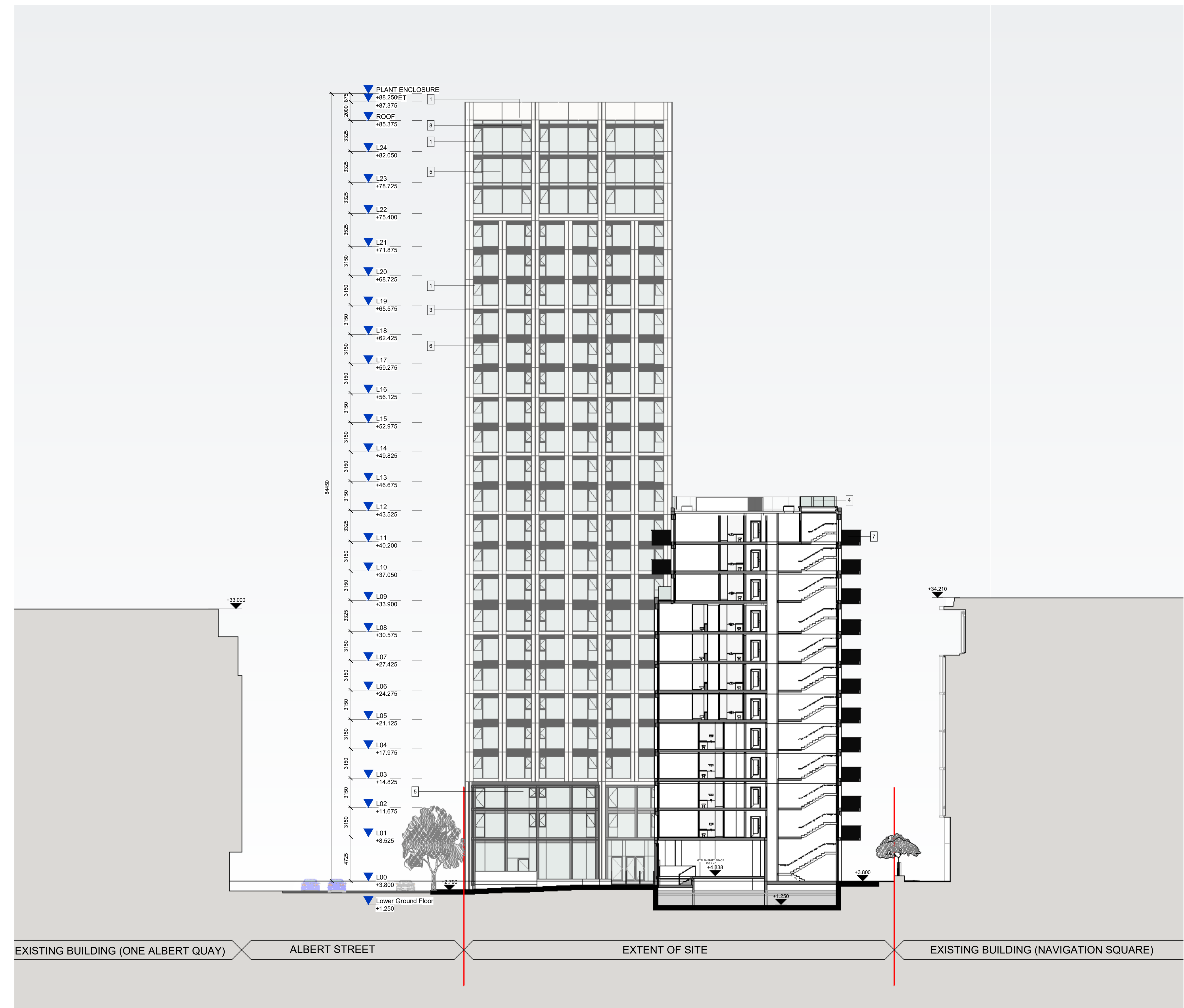
B-B SECTION B-B 1:200
