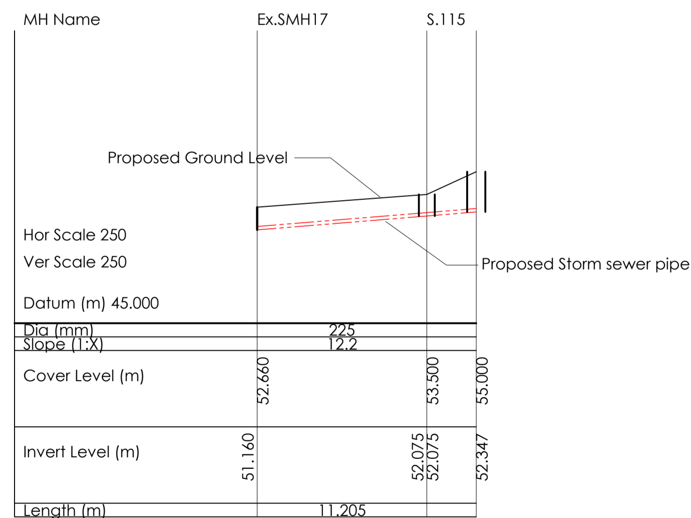
Longitudinal Storm Sewer Section MH's ex.SM17 - S.115 Scale: 1:250
