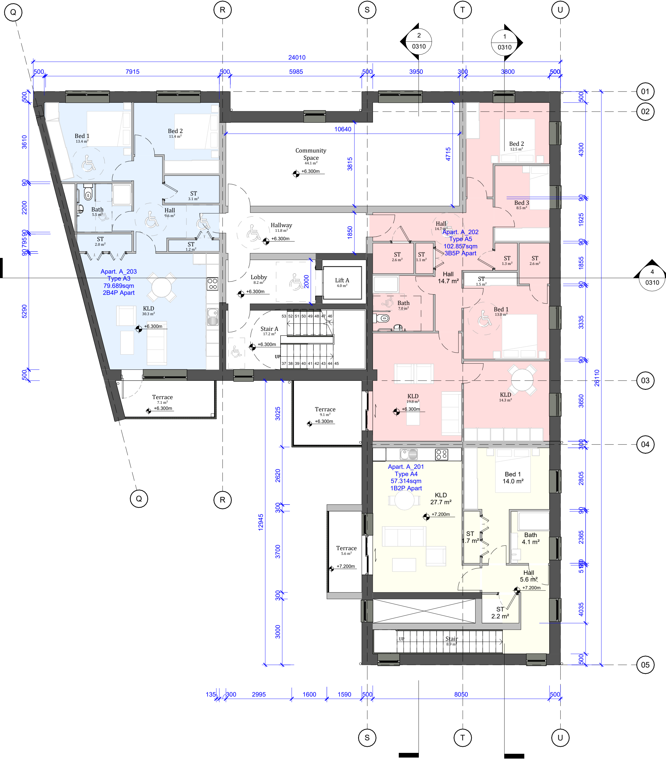
1 Level 02 - Block A 1 : 100
