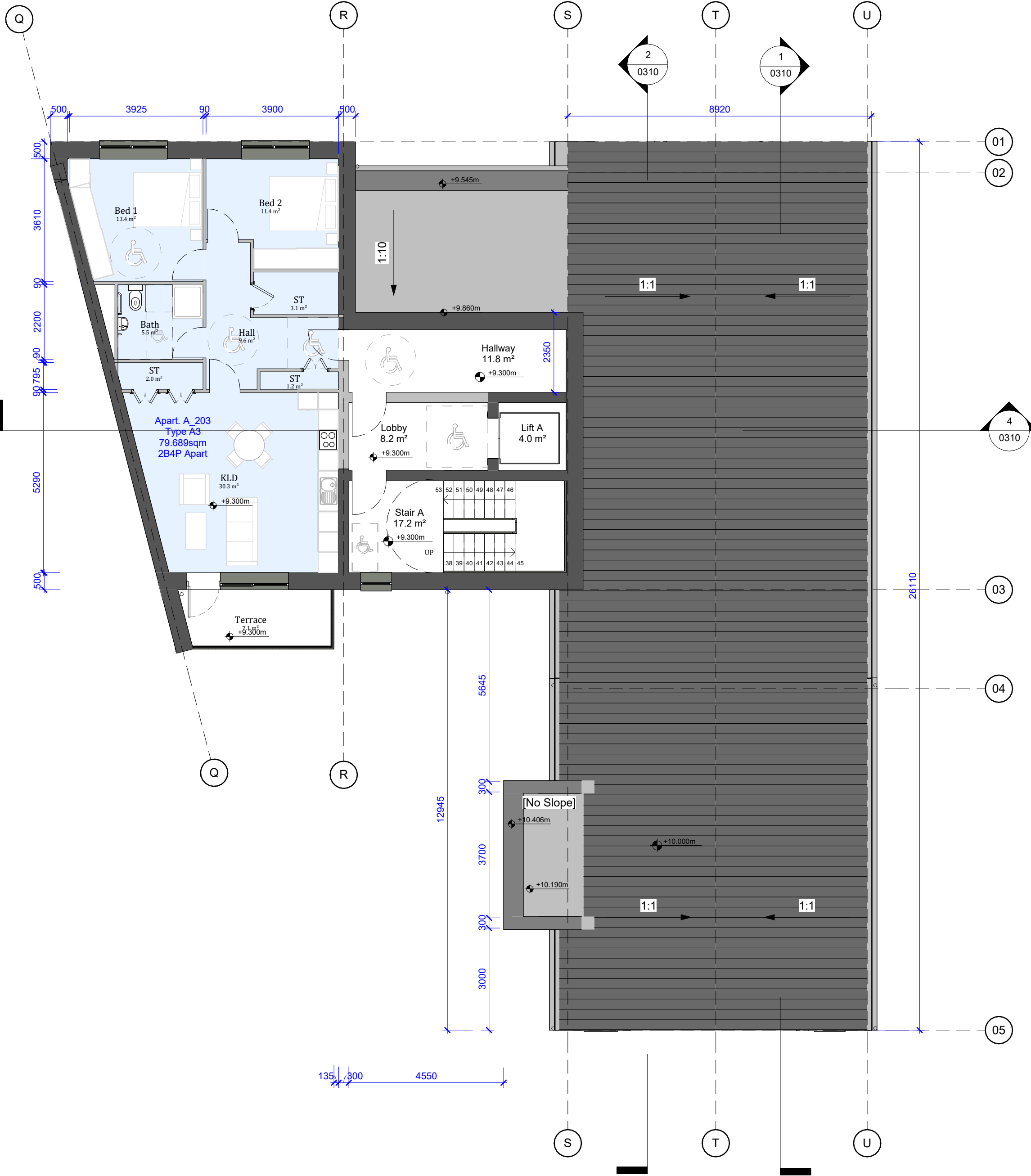
2 Level 03 - Block A 1 : 100
