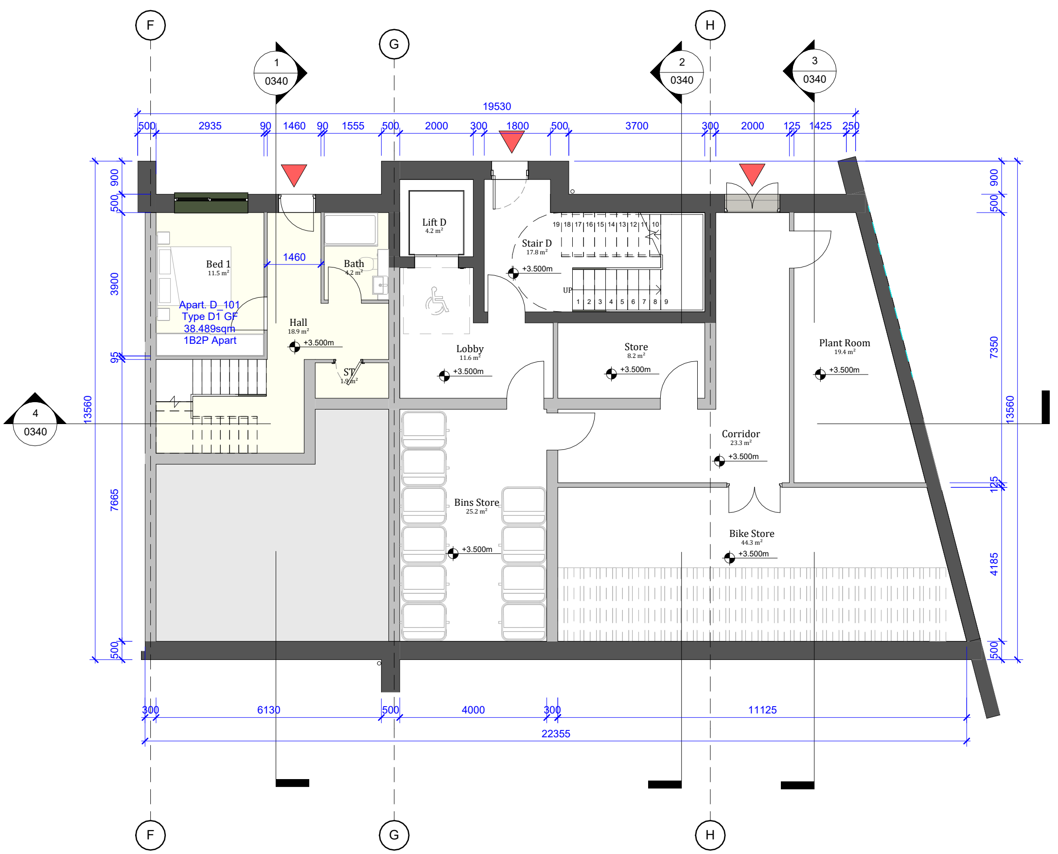
1 Level 01 - Block D 1 : 100
