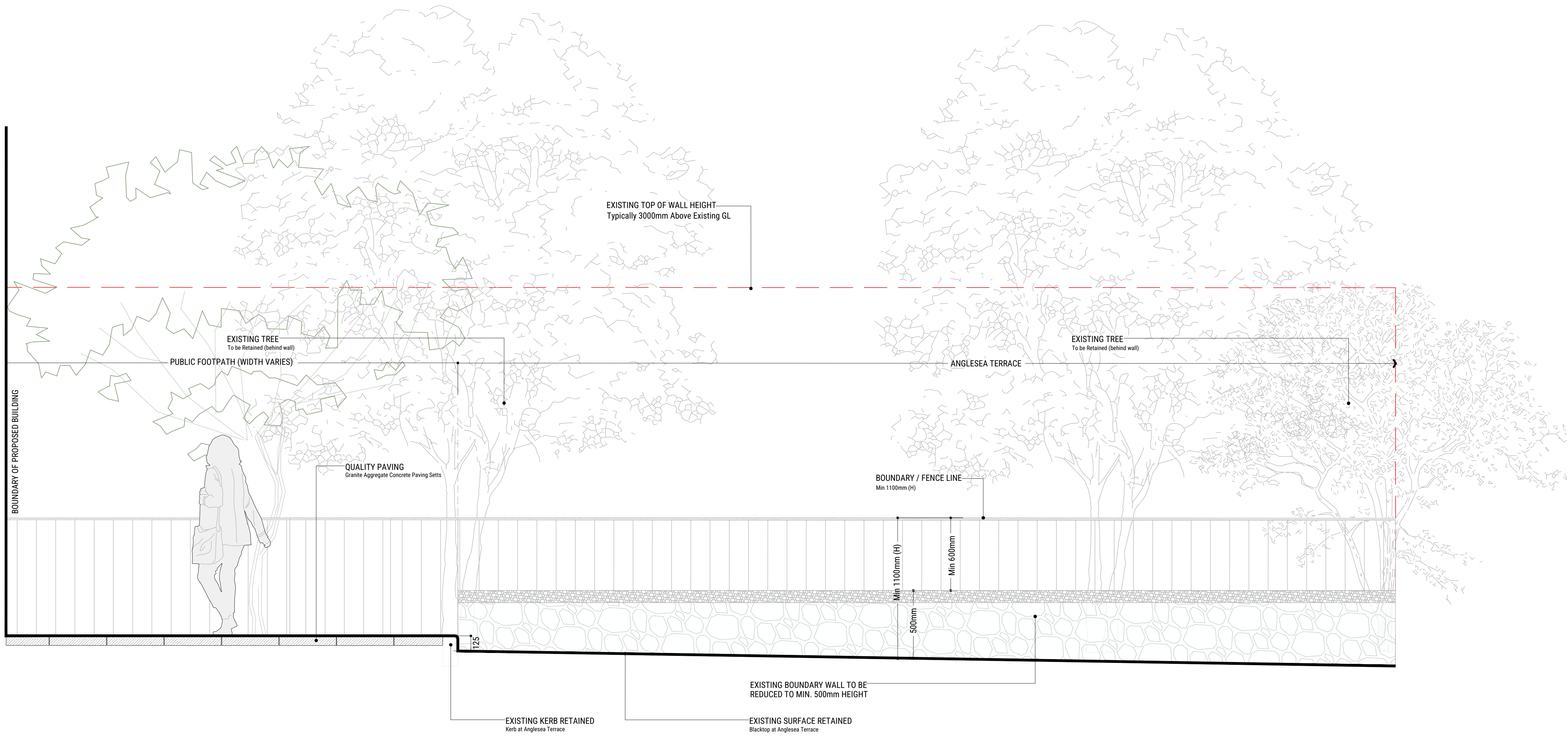
S Elevation S SCALE: 1:20 @ A1
