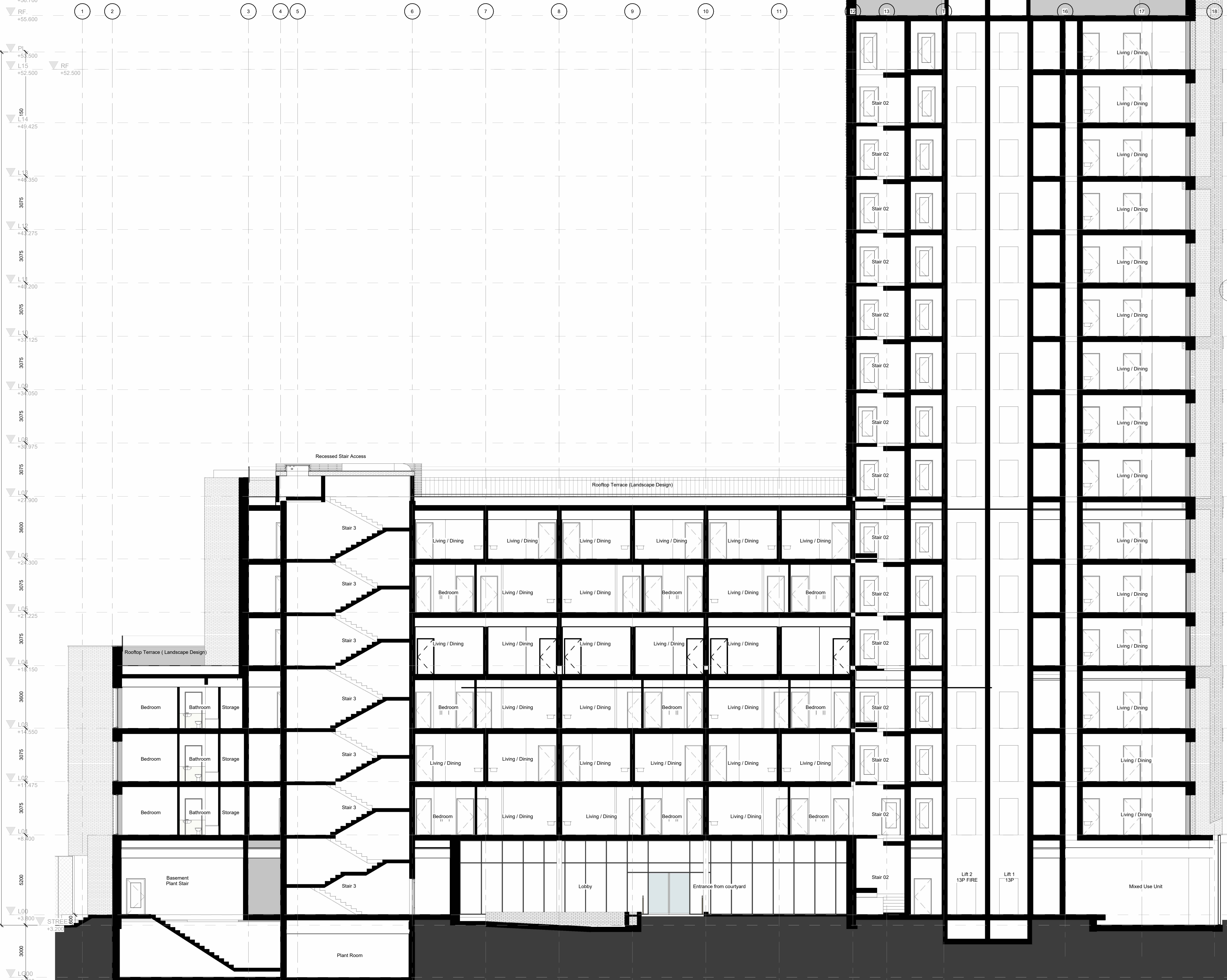
SECTION A-A 1 : 100
